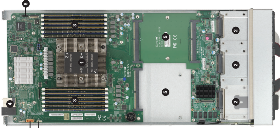
SBI-6419P-C3N Module Layout
