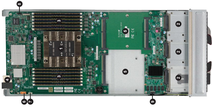
SBI-6119P-C3N Module Layout
