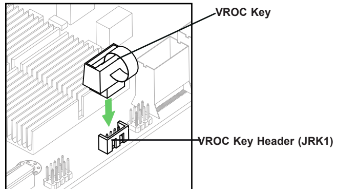
1. VROC RAID Key Header (JRK1)
